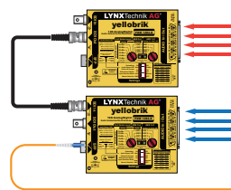
光ファイバー接続でのシステム
