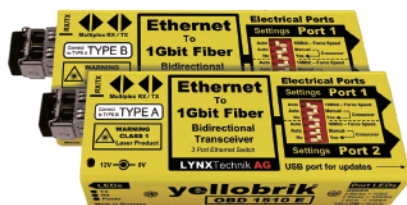
二台セット モデル 光ファイバー 1芯接続 WDM 機能内蔵
